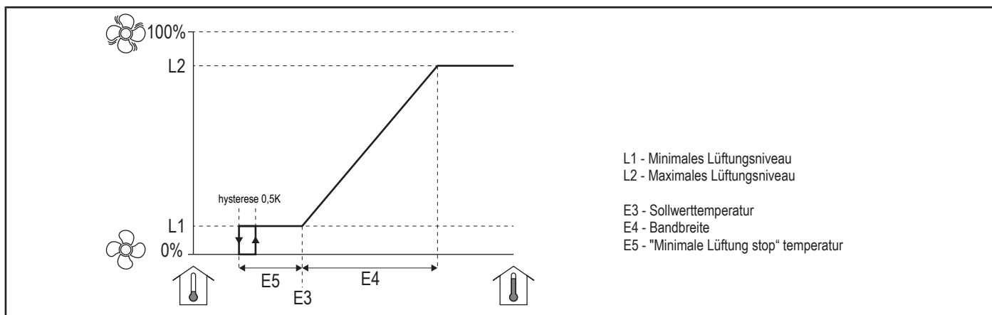
Abb. 2: Lüftungsniveau
