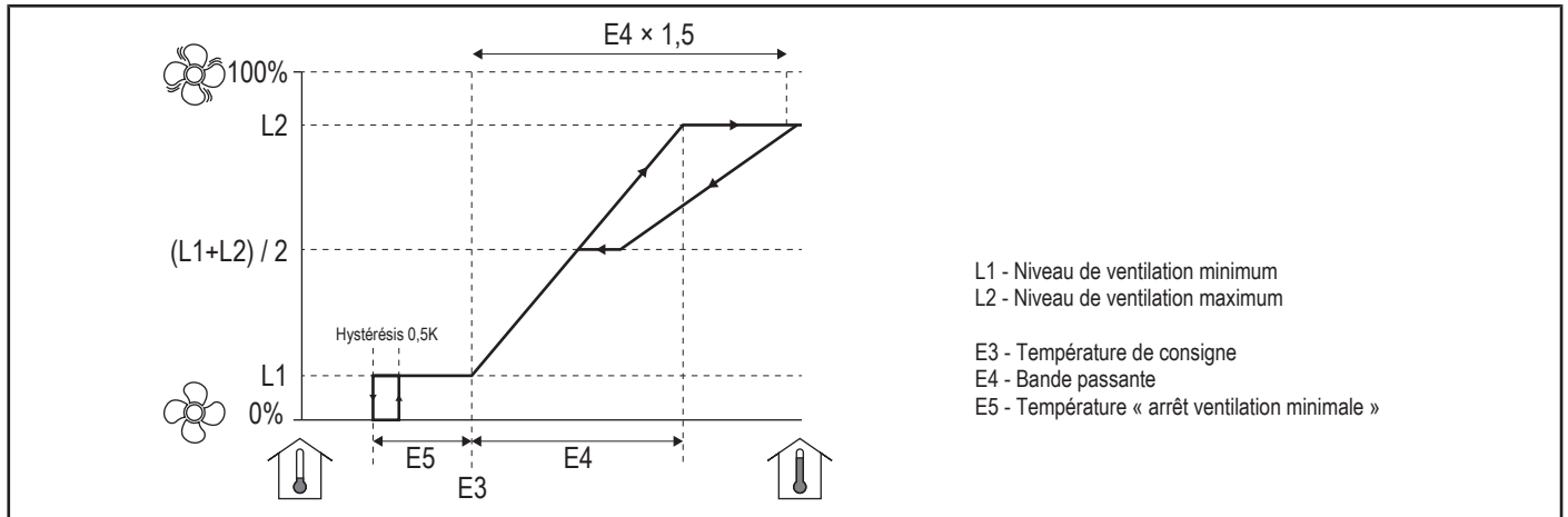
Fig. 4: Compensation de la bande passante
