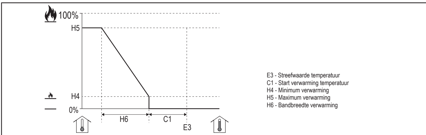
Afbeelding 7: Verwarming [0 - 10 V]
