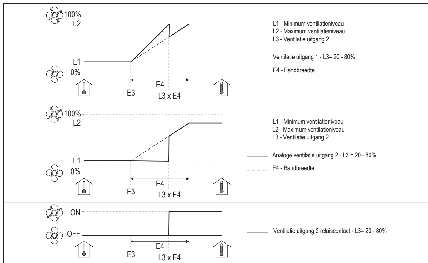
Afbeelding 3: Ventilatie uitgang 2 - [20 - 80%]
