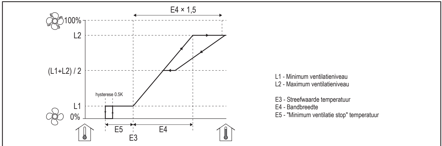
Afbeelding 4: Bandbreedtecompensatie
