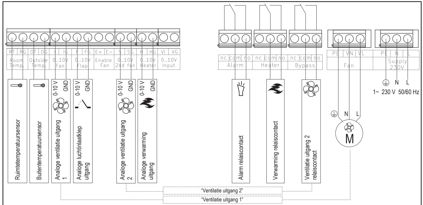
Afbeelding 1: Aansluitschema
