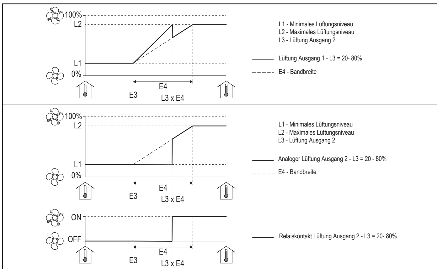
Abb. 3: Lüftung Ausgang 2 - [20 - 80%]
