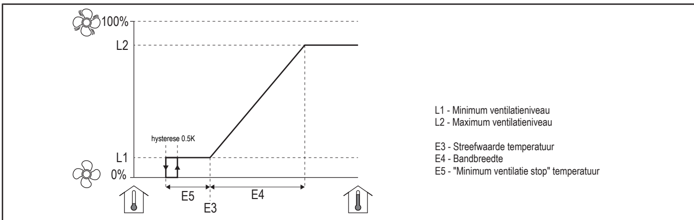
Afbeelding 2: Ventilatie niveau
