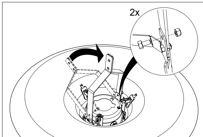
Fig. 3: Redressement du support
