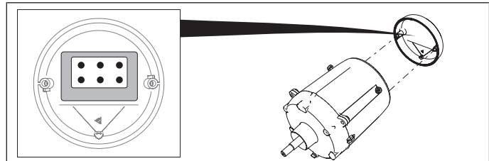
Afbeelding 10: Locatie van het aansluitschema
