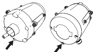
Ilustración 9: Ubicación de los agujeros de drenaje del condensado
