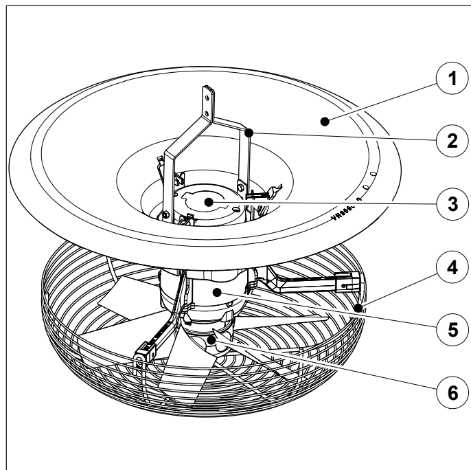
Abb. 1: V-FloFan Übersicht
