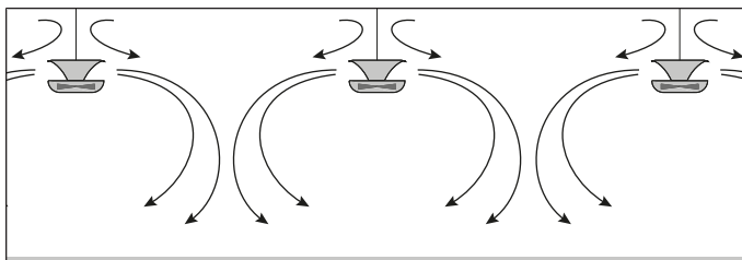
Abb. 2: Funktionsprinzip des VFloFan
