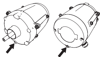
Afbeelding 9: Condensaatafvoergat locaties
