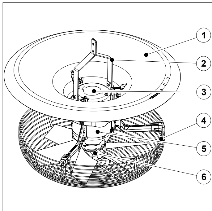
Afbeelding 1: V-FloFan overzicht
