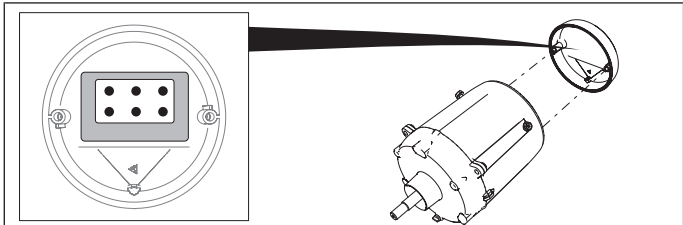
Ilustración 10: Localización del esquema de cableado
