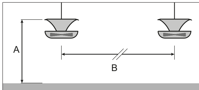
Fig. 4: V-FloFan position d'installation
