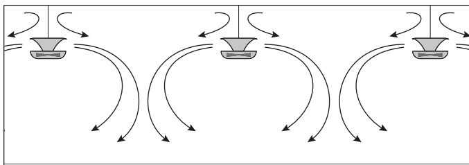
Fig. 2: Principe de fonctionnement VFloFan
