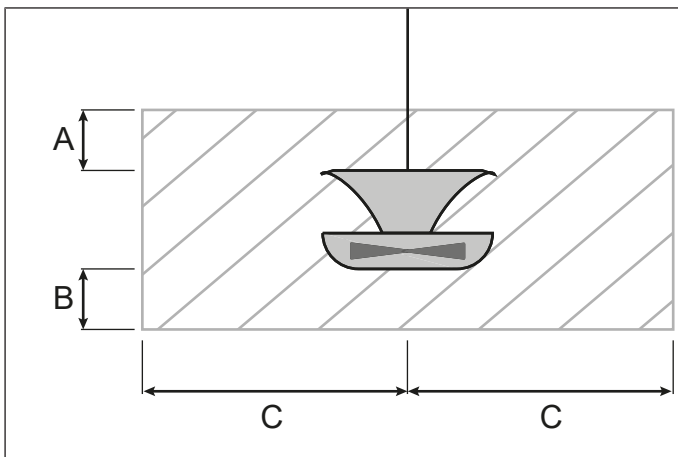
Abb. 5: V-FloFan hindernisfreier Bereich
