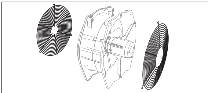
Ilustración 3: Juego de resguardos disponible opcionalmente
