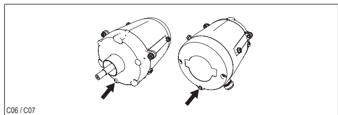
Fig. 5: Emplacement des trous de drainage du condensat
