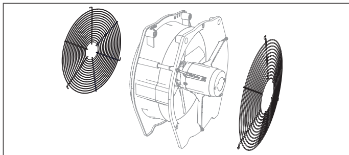
Afbeelding 3: Optioneel verkrijgbare set afschermingen
