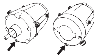
Abb. 5: Positionen der Kondensatablauflocher
